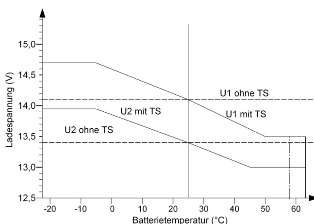
Ladeprogramm „MOTOR“ (FNFW), Kennlinie IU1oU2
